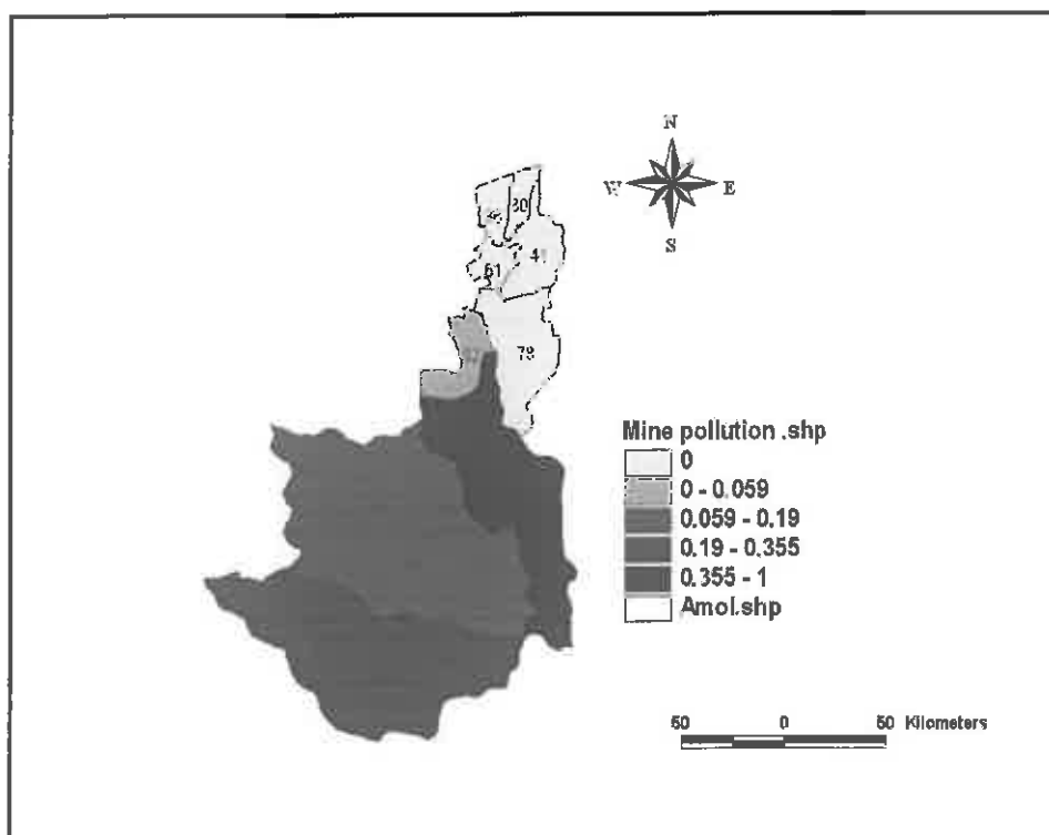
شکل ۵-۶- شدت نسبی بار وجود منابع آلاینده- معادن
