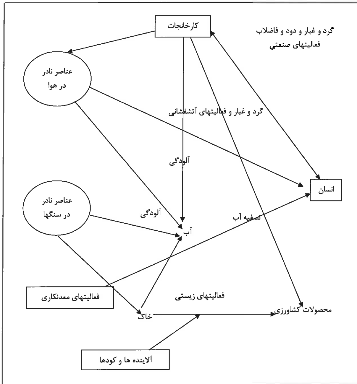
شکل ۲-۳- راه‌ها و فرآیندهایی که عناصر مختلف از طریق آنها به بدن انسان وارد می‌شوند (غضبان ۱۳۸۱، با
