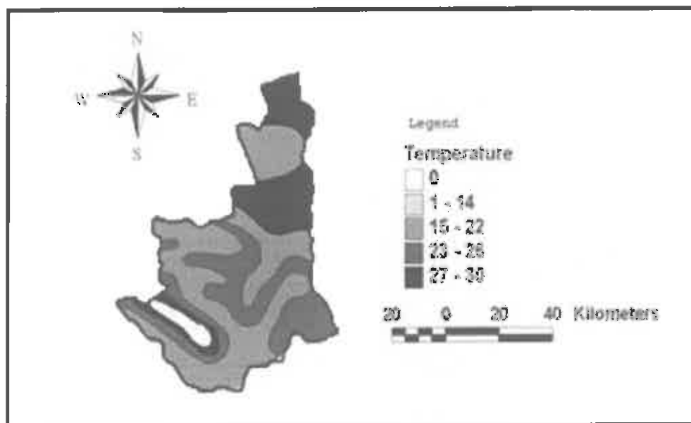
شکل ۷-۲ خطوط همدمای شهرستان آمل
