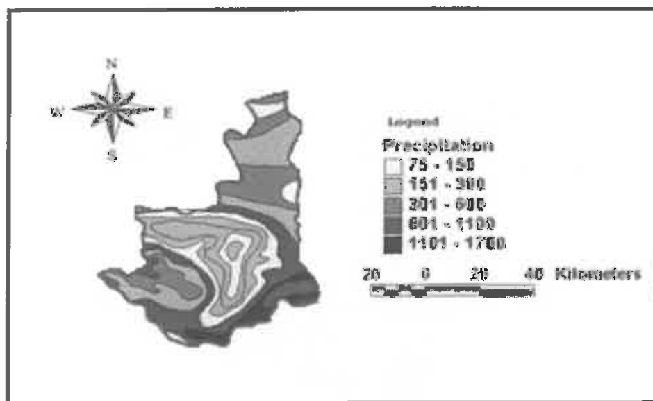
شکل ۶-۲- خطوط همبارش شهرستان آمل
