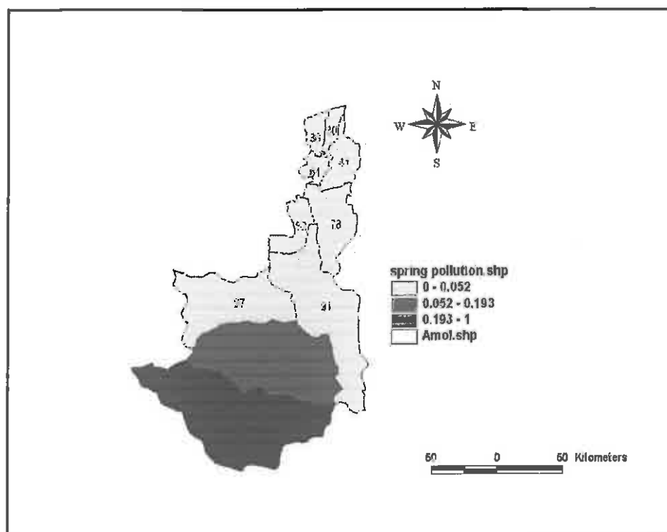
شکل ۴-۶- شدت نسبی بار وجود منابع آلاینده- چشمه های هیدروترمال
