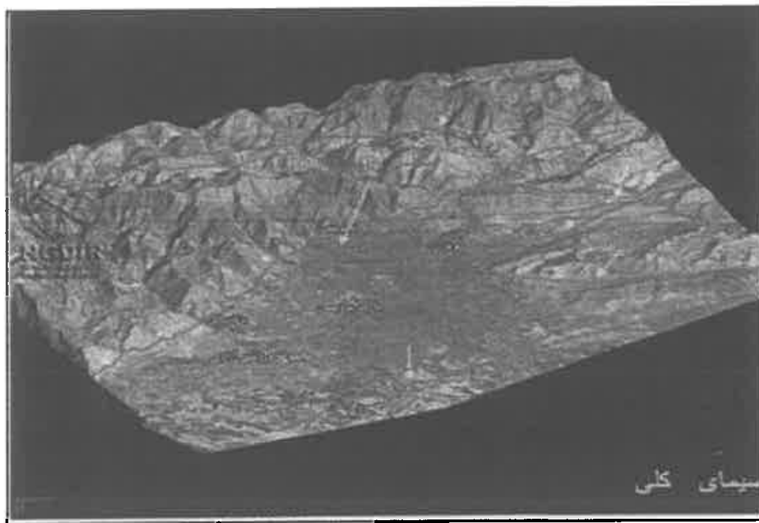
شکل ۵-۲- نمای سه بعدی از گسلهای مهم البرز مرکزی (اقتباس از سازمان زمین شناسی)
