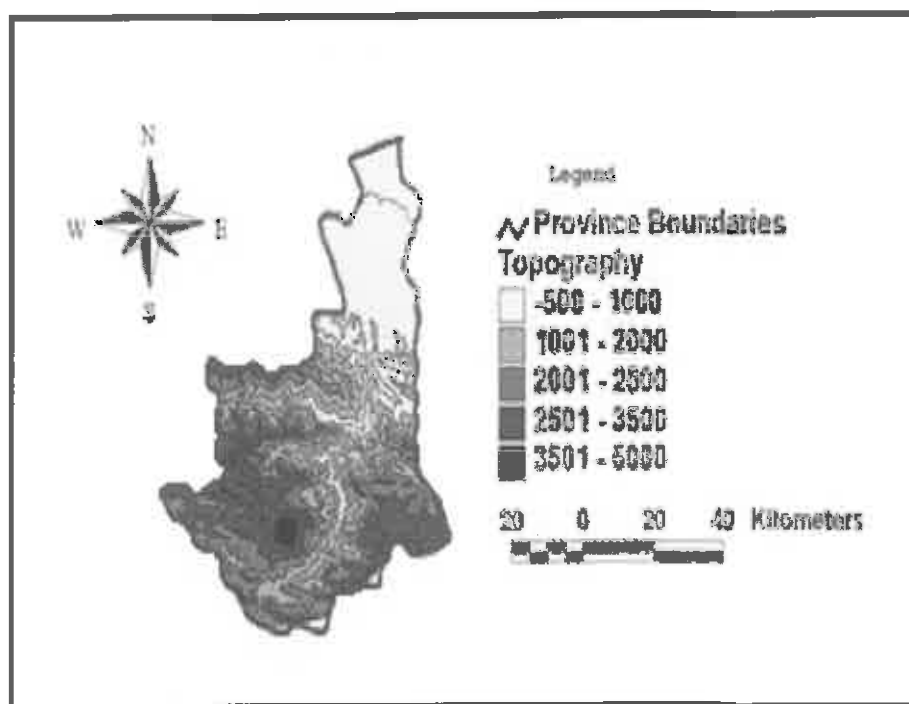
شکل ۳-۲- توپوگرافی شهرستان آمل
