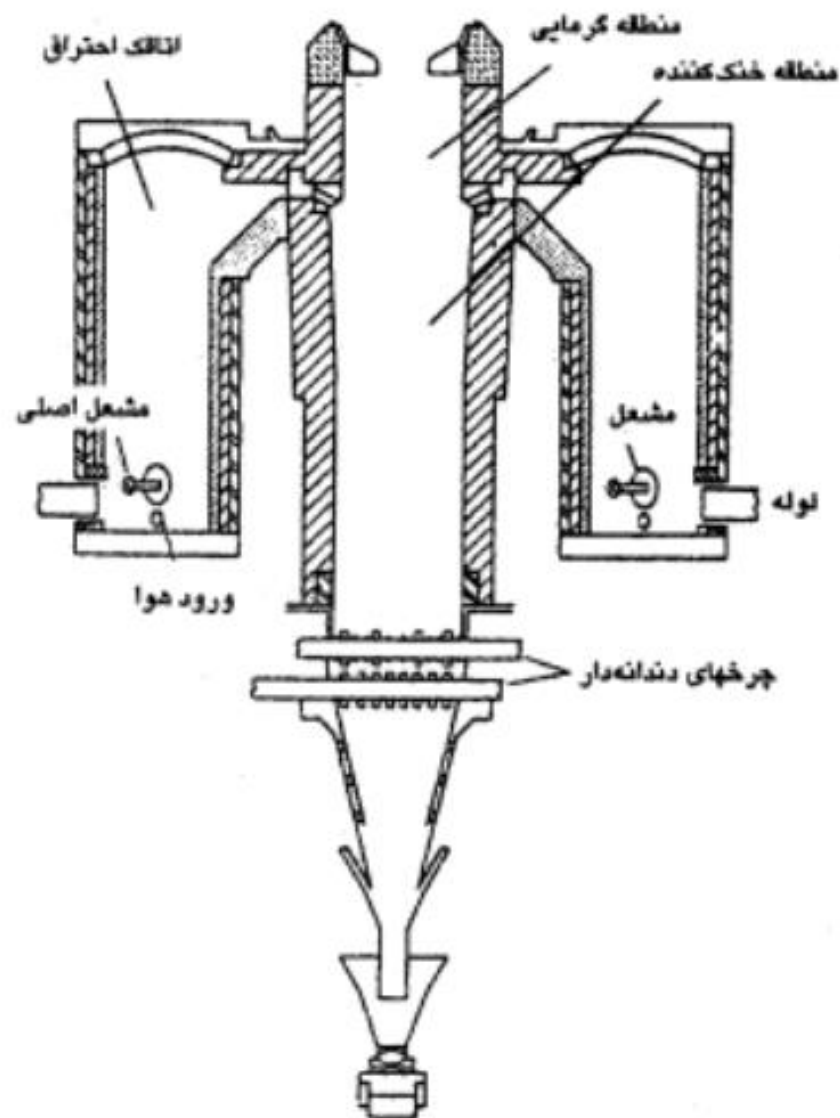
نمایی از کوره تنوره‌ای قائم
